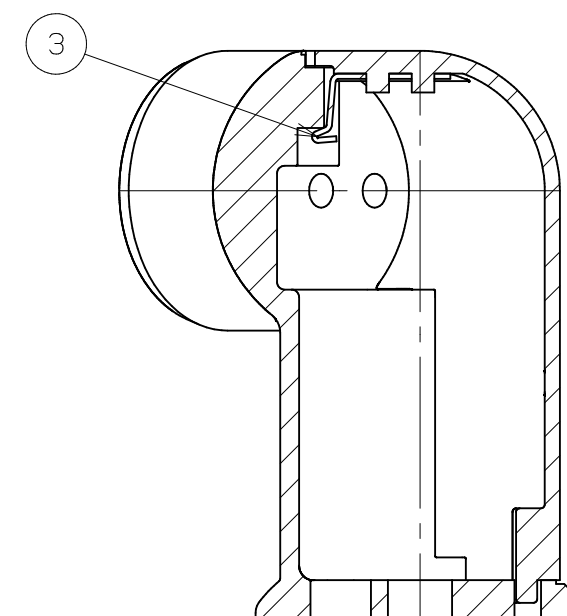
A-A断面図 尺度(1/1)
